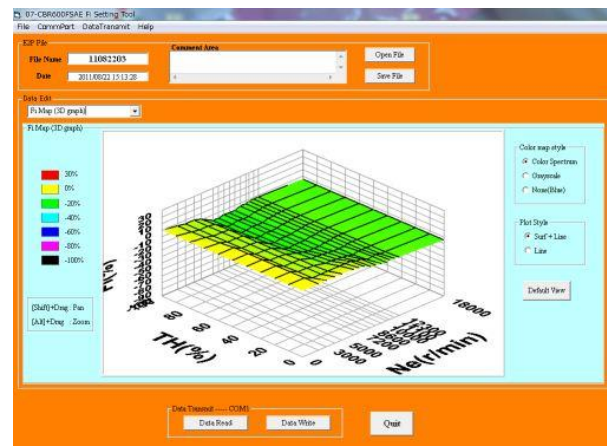
図3、燃調マップ
