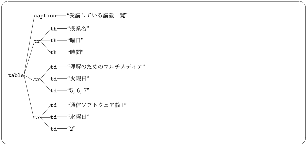
図 4.2 図 4.1 の構文木
