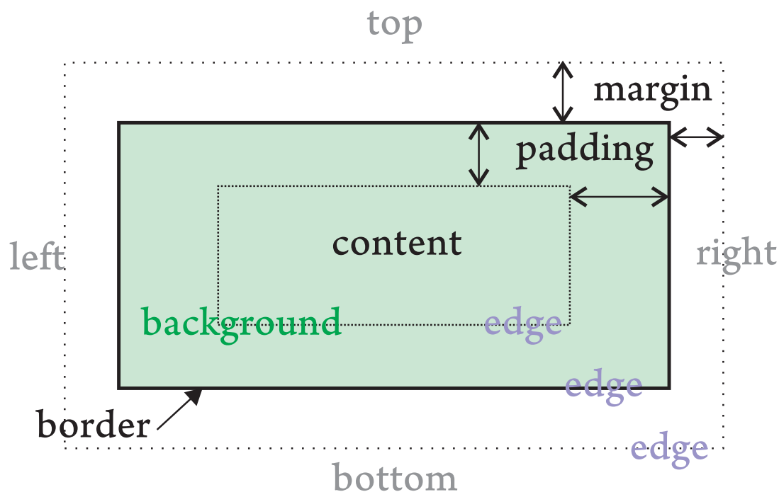
図 5.3 CSS のボックスモデル
