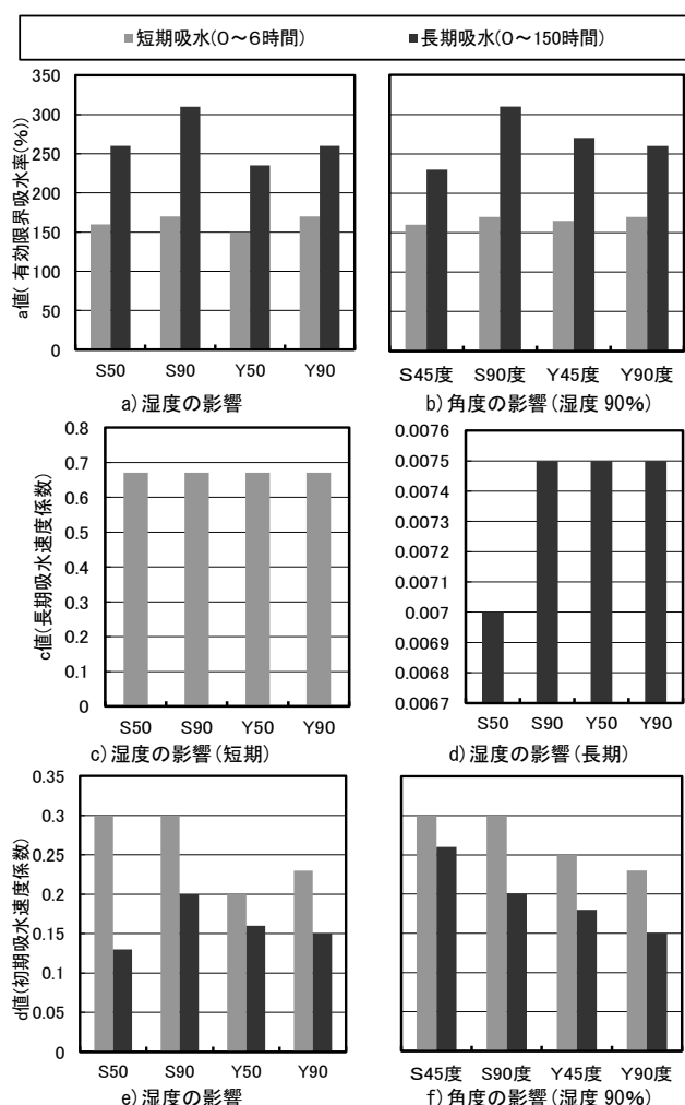
図 4 吸水試験結果による理論式定数の特性 (b 値は 1 で一定)
