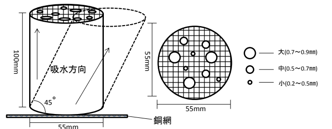
1) 試験体側面図(90°・45°) 2) 試験体断面図 3) 茅素材の直径区分 a) 吸水試験体概要図
