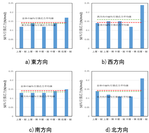
図 5 シーリング材の引張試験の 50%引張応力の結果
