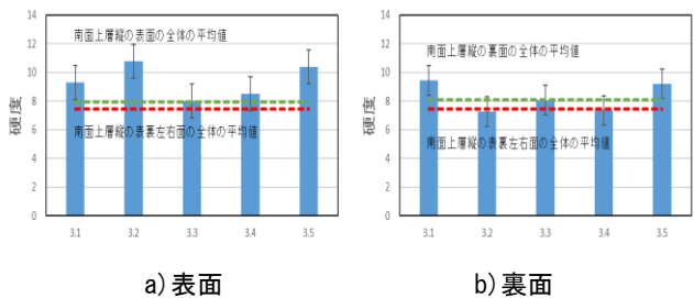
図 7 南面上層縦のシーリング材の表面と裏面の結果の比較
