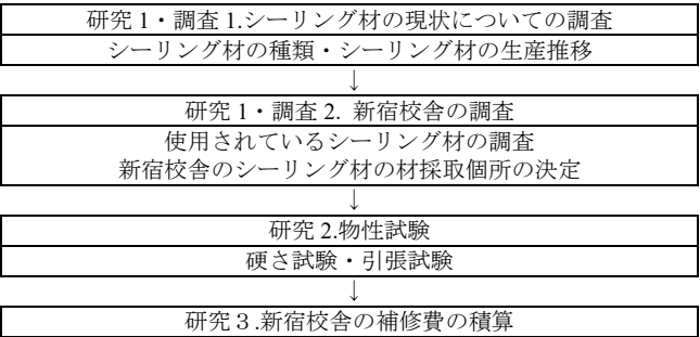
図 1 研究の流れ
