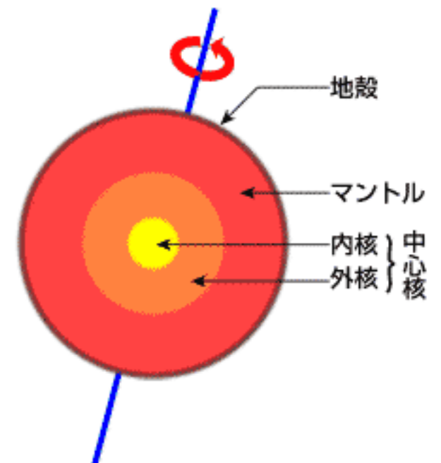
鉄の中心核が回転して磁石ができる
