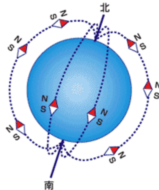
地球は大きな磁石になっている
