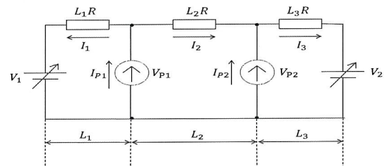
図1 等価回路図(回生2列車)
