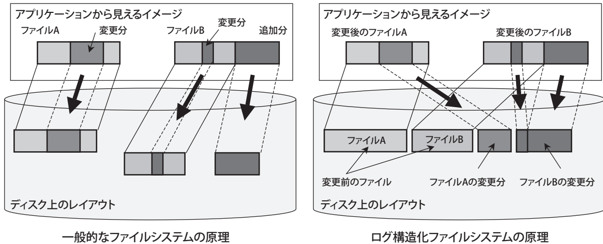
図-2 ログ構造化ファイルシステム
