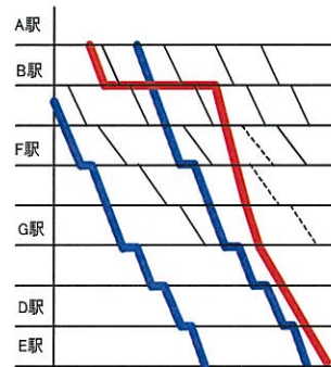
図4. 緩行列車のみ待避時
